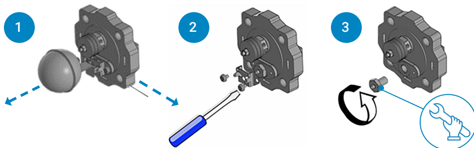
Рисунок 11. Последовательность проведения ремонтных работ конденсатоотводчика.
