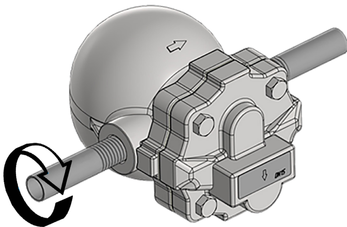
Рисунок 7. Визуальное изображение монтажа конденсатоотводчика с резьбовым присоединением.
