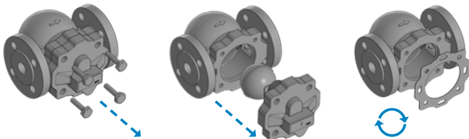
Рисунок 10. Последовательность проведения ремонтных работ конденсатоотводчика.
