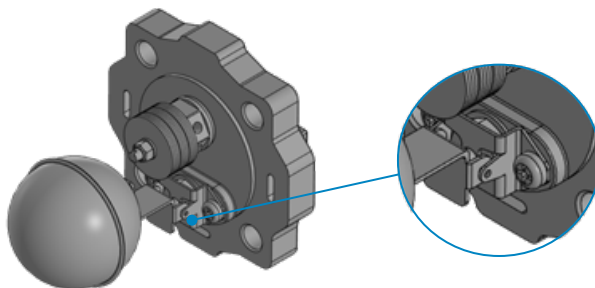
Рисунок 13. Установка поплавка.
