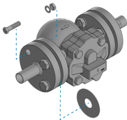
Рисунок 8. Визуальное изображение монтажа конденсатоотводчика с фланцевым присоединением.
