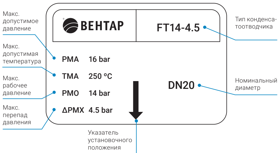
Рисунок 5. Описание элементов маркировочной таблички конденсатоотводчика FT14.
